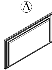
x1 Headboard panel x1 Tête de lit x1 Panel de la cabecera
