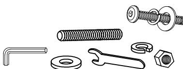
x1 RS860DJ-272-HWKIT-Hardware kit list* Liste des pièces de quincaillerie Lista del kit de materiales
