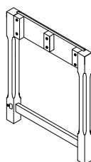
x1 RS862DJ-113- LEGR -Right leg * Patte de droite Pata derecha
